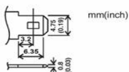
F1 (FASTON TAB NO. 187)
